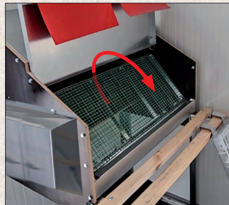
AUTOMATISCHER NESTAUSTRIEB
